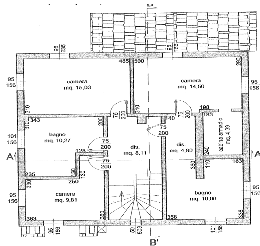
Piano Primo
